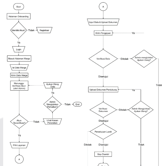
Gambar 2 Alur Kerja Aplikasi Warga
