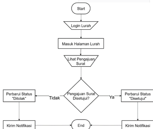
Gambar 4 Alur Kerja Aplikasi Lurah
