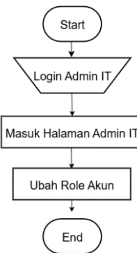
Gambar 5 Alur Kerja Aplikasi Admin IT
