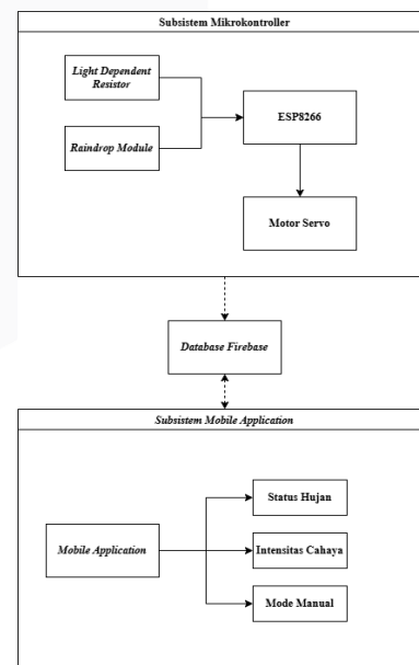
GAMBAR 1 (Gambar Arsitektur Sistem)
