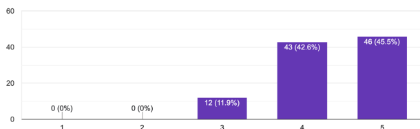
GAMBAR 16
