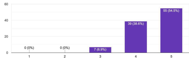
GAMBAR 17
