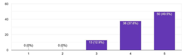
GAMBAR 13
