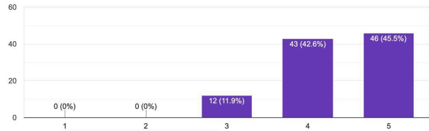
GAMBAR 9
