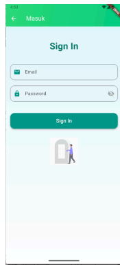
GAMBAR 4 (Halaman Login)
