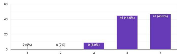
GAMBAR 18
