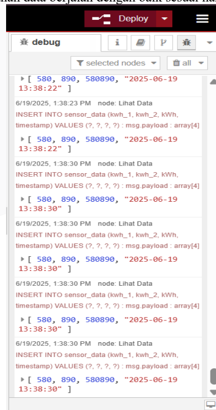
Gambar 4. 2 Debug /keluaran dari flow Node-RED
