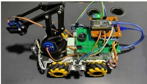
Gambar 9 Hasil Akhir Implementasi Robot
