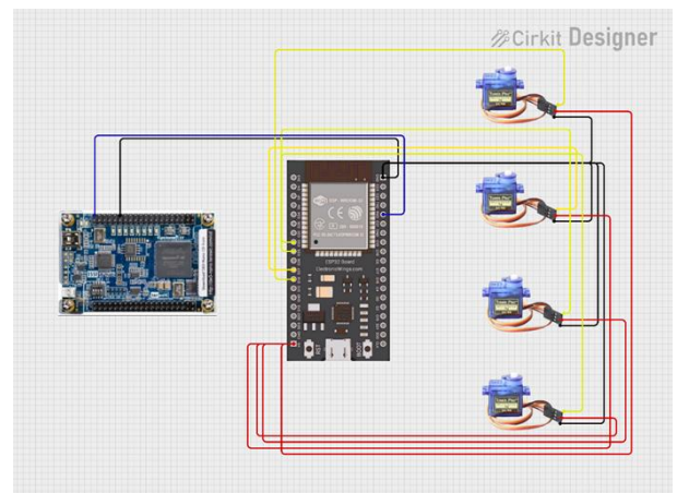
GAMBAR 6 Skematik Penggerakan Robot Lengan
