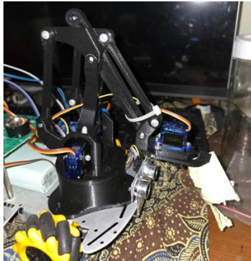
Gambar 10 Robot Lengan dengan Sampah
