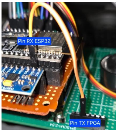
GAMBAR 8 Hasil Implementasi ESP32 dengan FPGA
