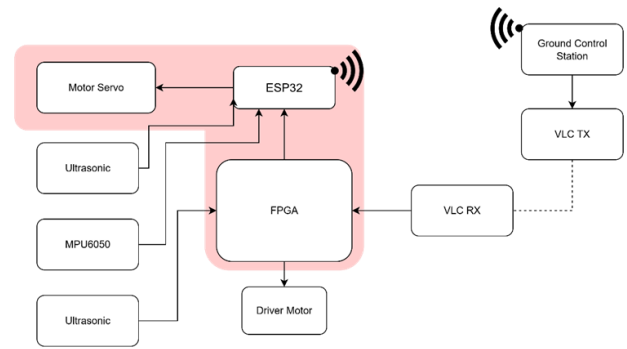
Gambar 2 Blok Diagram Sistem
