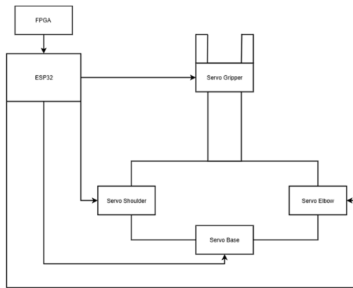
Gambar 4 Model Sistem Penggerak Robot Lengan
