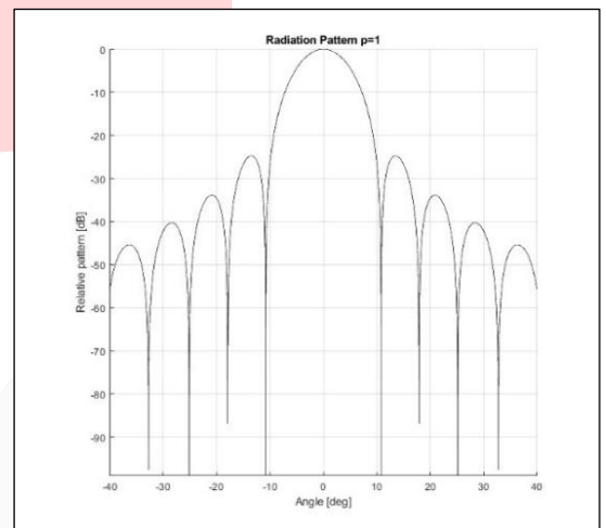
Gambar 7 Polaradiasi
