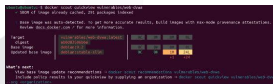
Gambar 7. Pemindaian Image Docker
