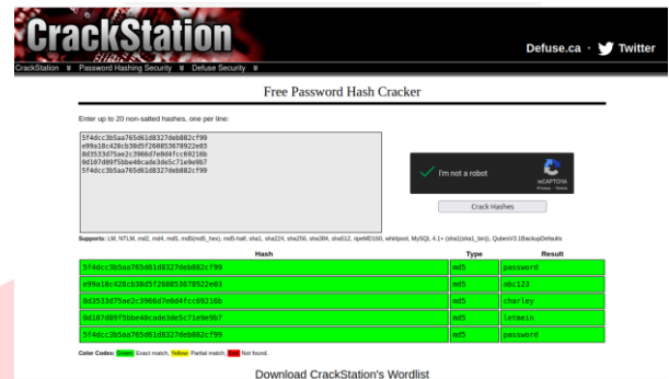
Gambar 15. Crackstation Memecahkan Hash Password
