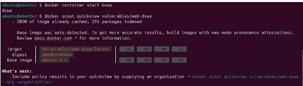
Gambar 9. Pemindaian Image Docker Setelah Run
