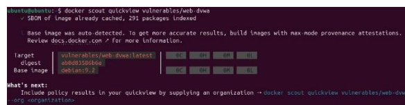
Gambar 8. Pemindaian Image Docker Sebelum Run
