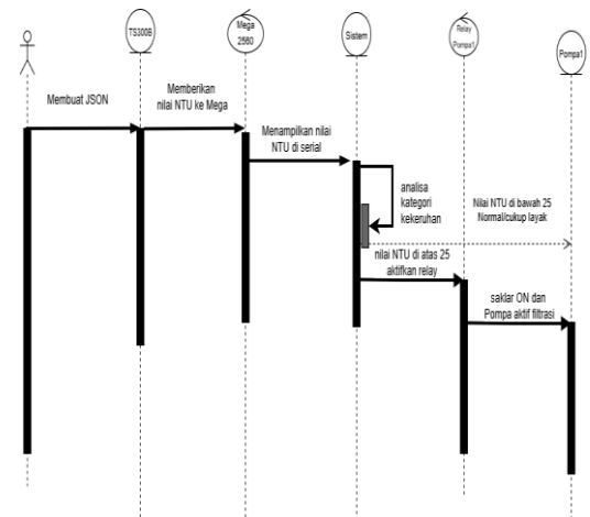
Gambar 1 Sequence Diagram parameter NTU
