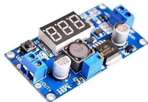
Gambar 10 Modul LM2596
