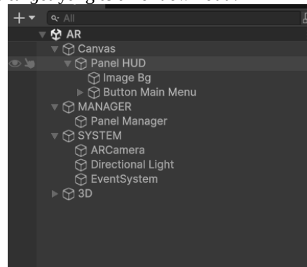
GAMBAR 11 Hierarchy KameraAR
