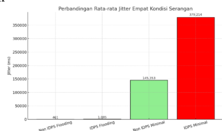
GAMBAR 31 (PERBANDINGAN NILAI JITTER PADA SETIAP PENGUJIAN)
