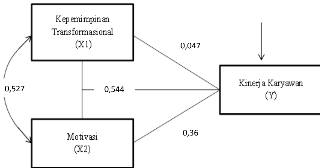
Gambar 3 Diagram Analisis Jalur
