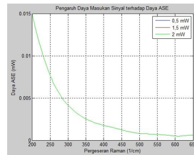
Gambar 4.10 Pengaruh daya masukan sinyal terhadap daya derau ASE
