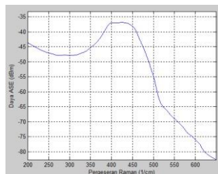
Gambar 4.19 Hasil peredaman (perataan) derau ASE dengan menggunakan filter FBG
