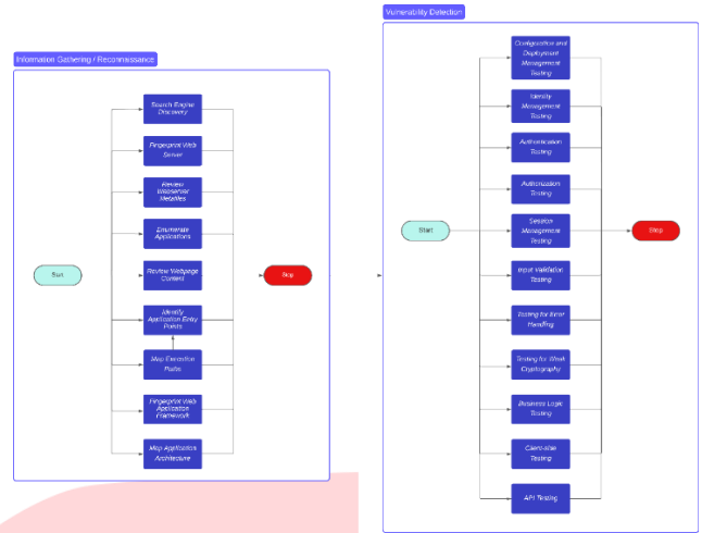
Gambar 4. Tahapan Metodologi OWASP WSTG
